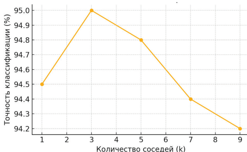
Рисунок 1 - Зависимость точности классификации от числа ближайших соседей k
